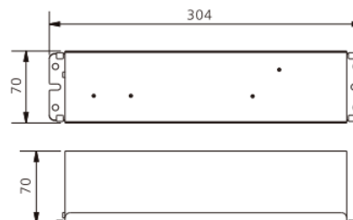
JLEB-16L-US JLEB-20L-US
